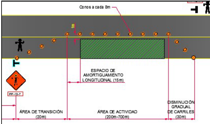
Figura 6. Longitudes en planos de las distancias de transición para zonas de 40 KPH.
