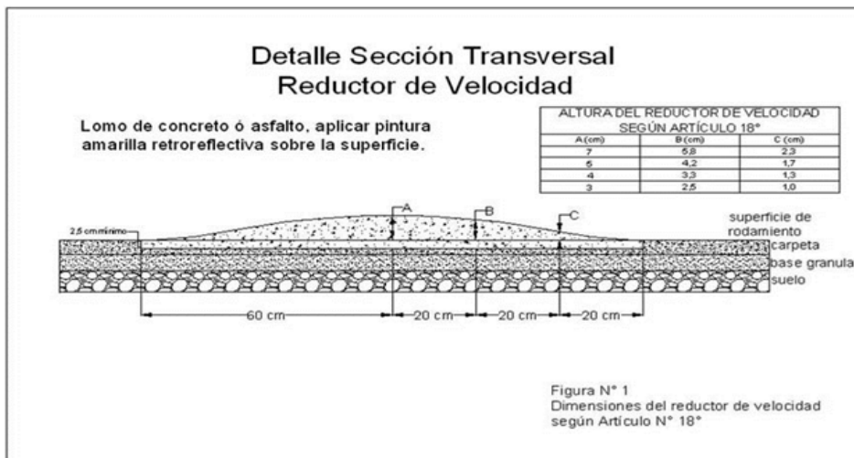
Figura N° 8 Corte típico de reductor de velocidad
