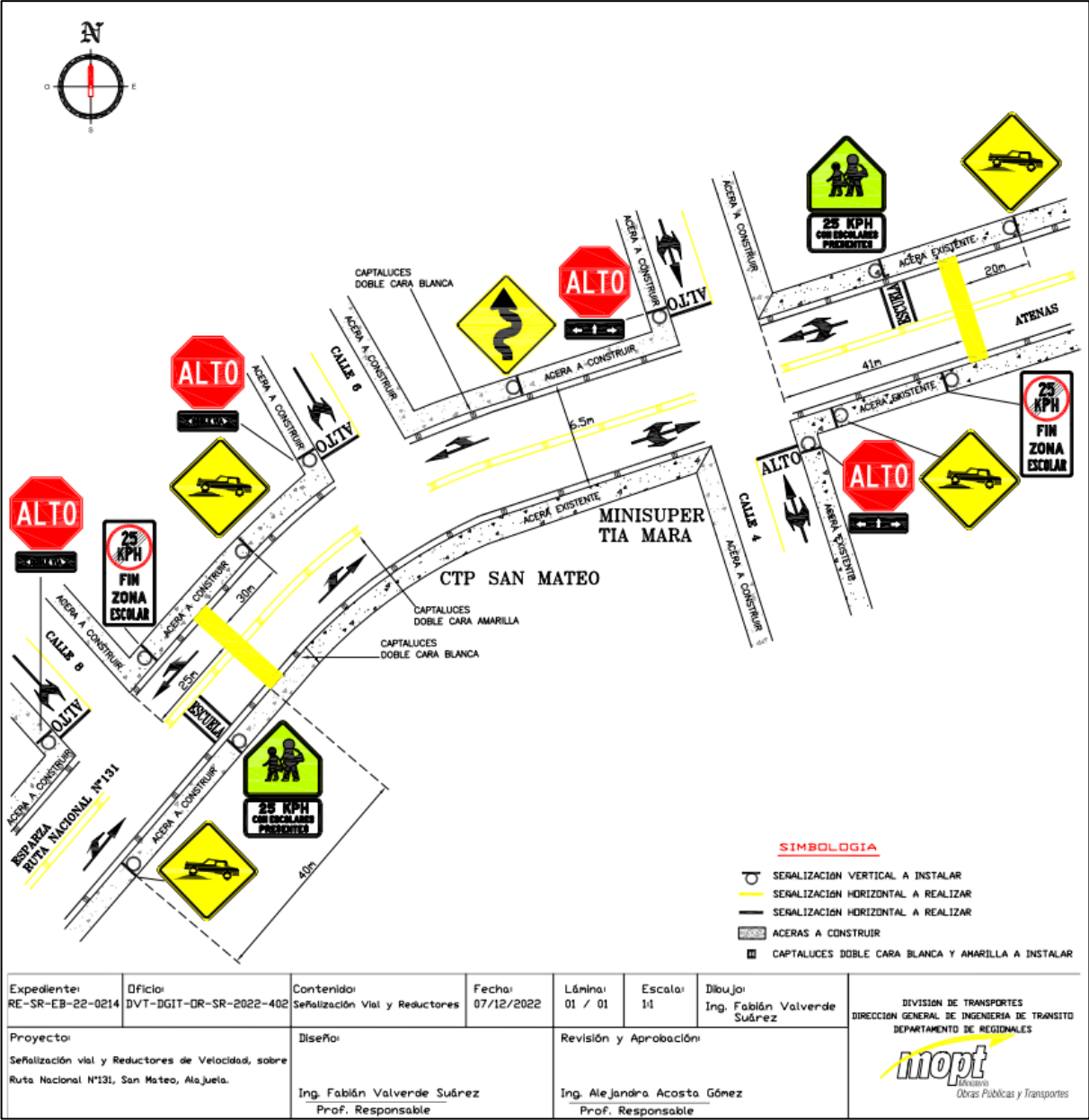
Figura N° 9. Croquis diseño señalamiento vial
