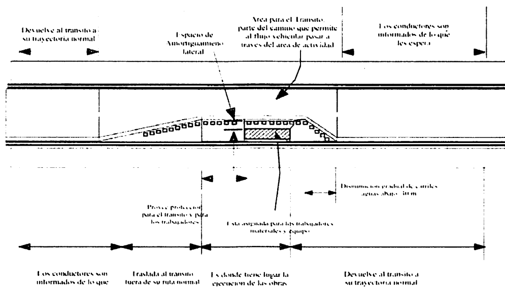
Figura 2. Componentes de las zonas de control de tránsito temporal.
