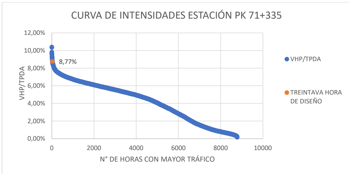
Gráfica 20: Curva de intensidades para obtención de Hora Treinta de Diseño de Estación 71+335
