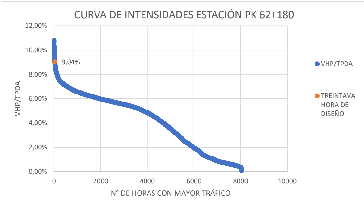
Gráfica 19: Curva de intensidades para obtención de Hora Treinta de Diseño de Estación 62+180
