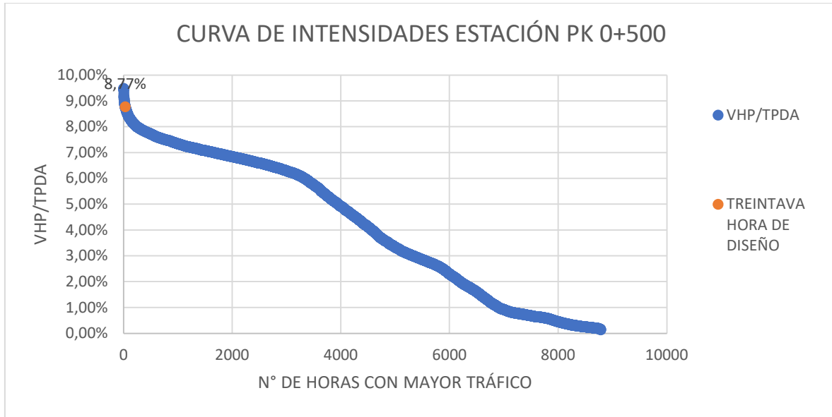
Gráfica 10: Curva de intensidades para obtención de Hora Treinta de Diseño de Estación 0+500
