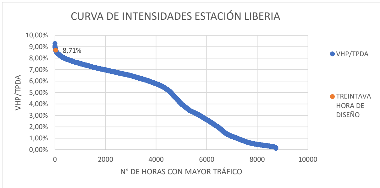
Gráfica 6: Curva de intensidades para obtención de Hora Treinta de Diseño de Estación Liberia
