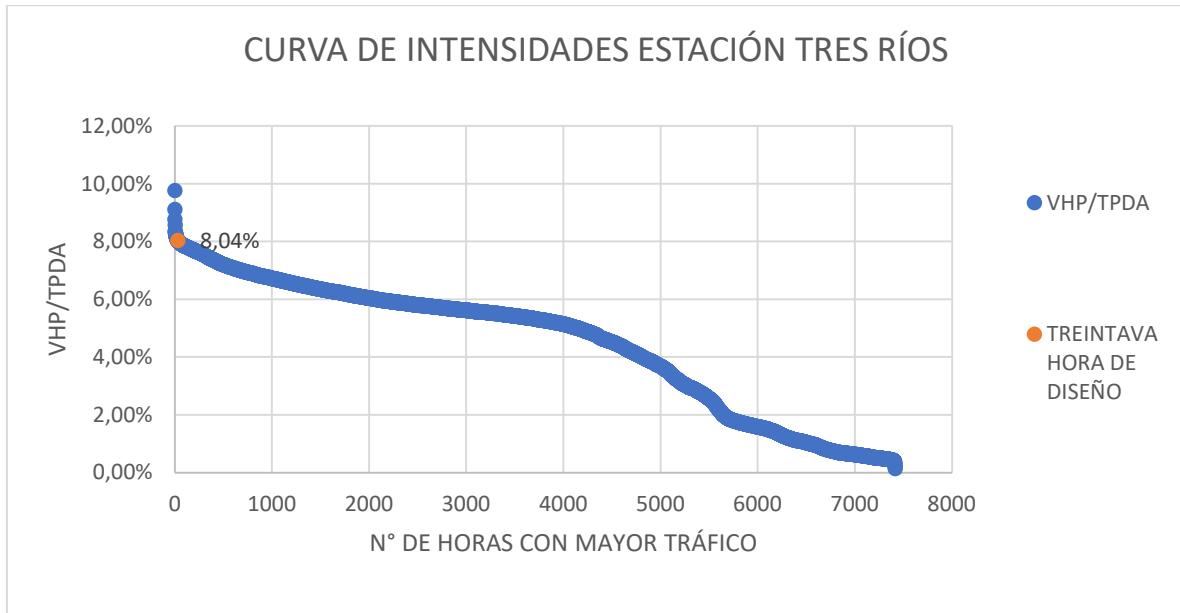
Gráfica 2: Curva de intensidades para obtención de Hora Treinta de Diseño de Estación Tres Ríos
