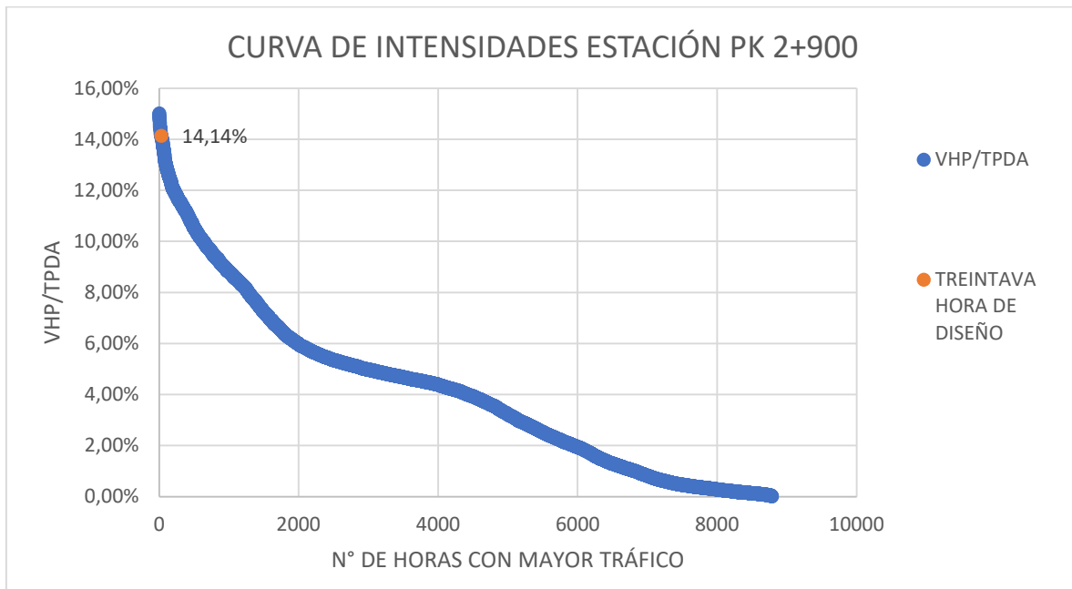
Gráfica 11: Curva de intensidades para obtención de Hora Treinta de Diseño de Estación 2+900
