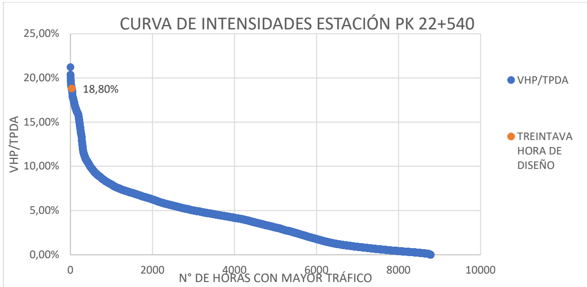
Gráfica 14: Curva de intensidades para obtención de Hora Treinta de Diseño de Estación 22+540
