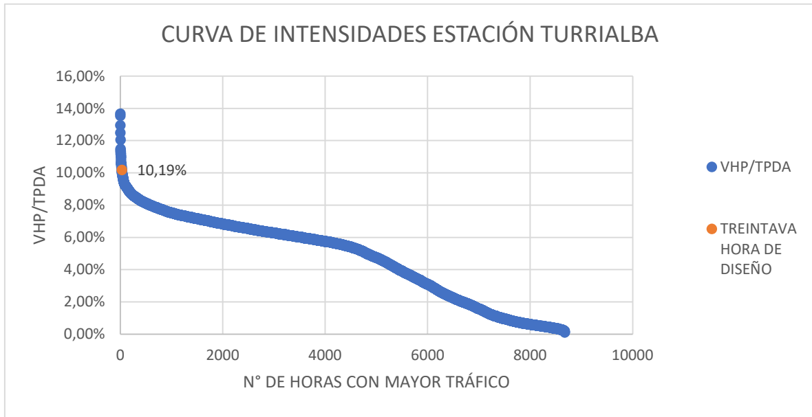
Gráfica 4: Curva de intensidades para obtención de Hora Treinta de Diseño de Estación Turrialba
