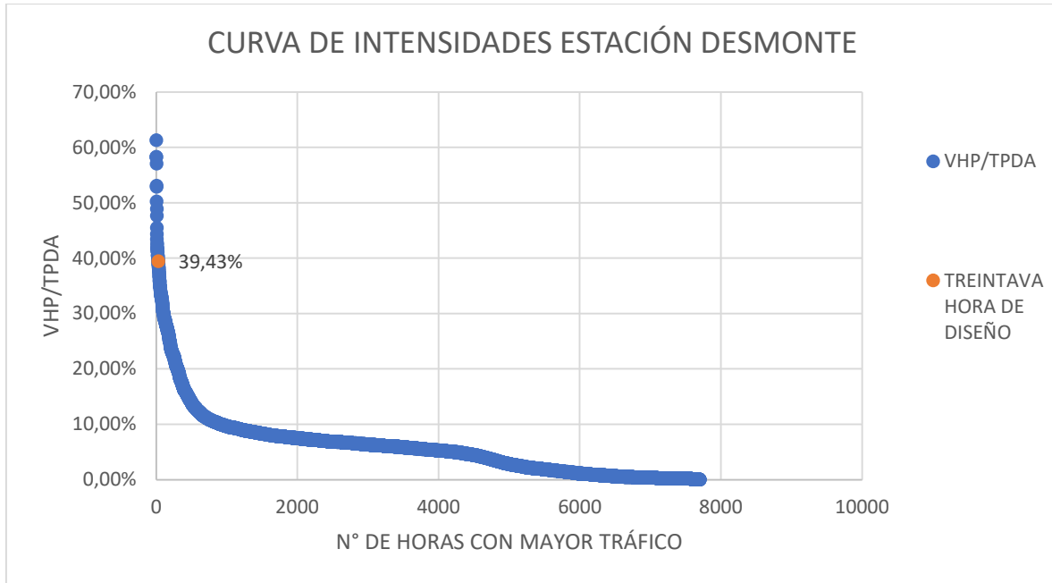
Gráfica 9: Curva de intensidades para obtención de Hora Treinta de Diseño de Estación Desmonte
