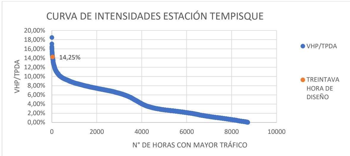
Gráfica 5: Curva de intensidades para obtención de Hora Treinta de Diseño de Estación Tempisque
