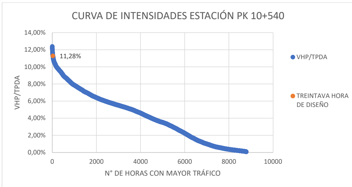
Gráfica 13: Curva de intensidades para obtención de Hora Treinta de Diseño de Estación 10+540
