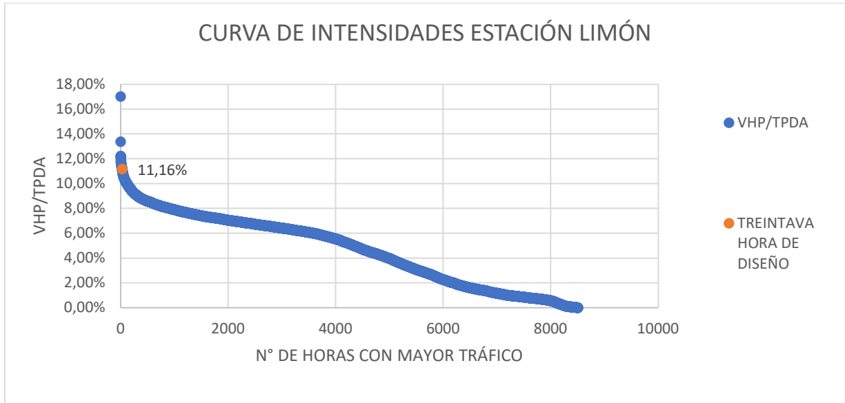
Gráfica 3: Curva de intensidades para obtención de Hora Treinta de Diseño de Estación Limón
