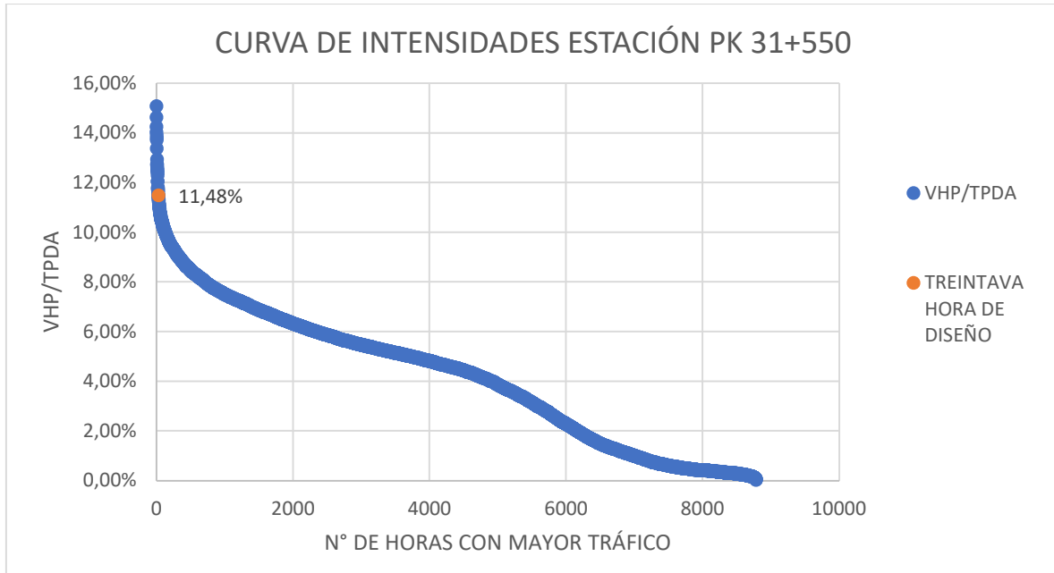
Gráfica 16: Curva de intensidades para obtención de Hora Treinta de Diseño de Estación 31+550
