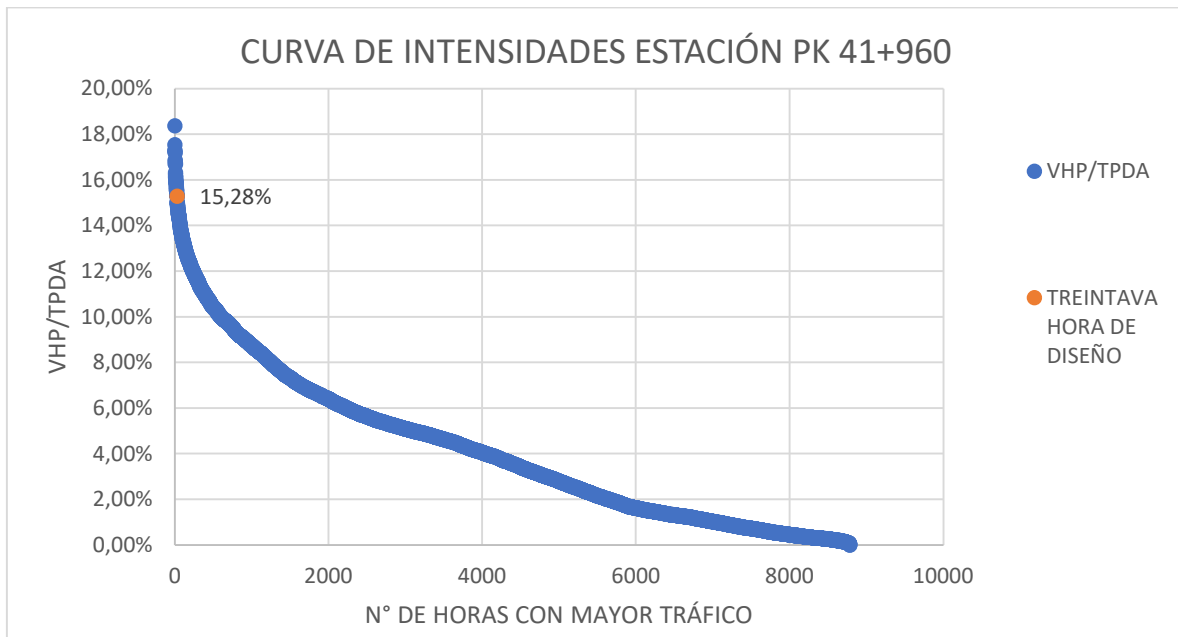
Gráfica 17: Curva de intensidades para obtención de Hora Treinta de Diseño de Estación 41+960
