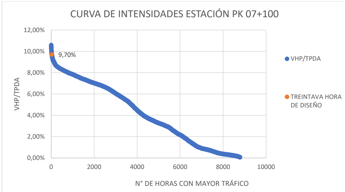
Gráfica 12: Curva de intensidades para obtención de Hora Treinta de Diseño de Estación 7+100
