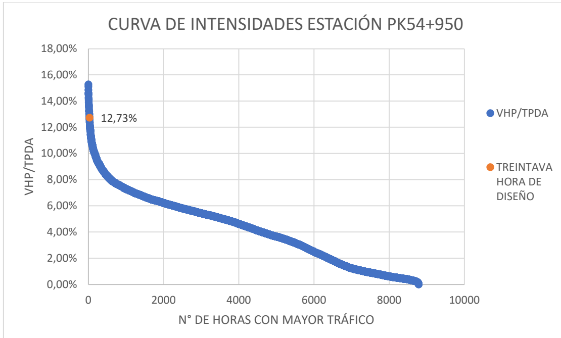
Gráfica 18: Curva de intensidades para obtención de Hora Treinta de Diseño de Estación 54+950
