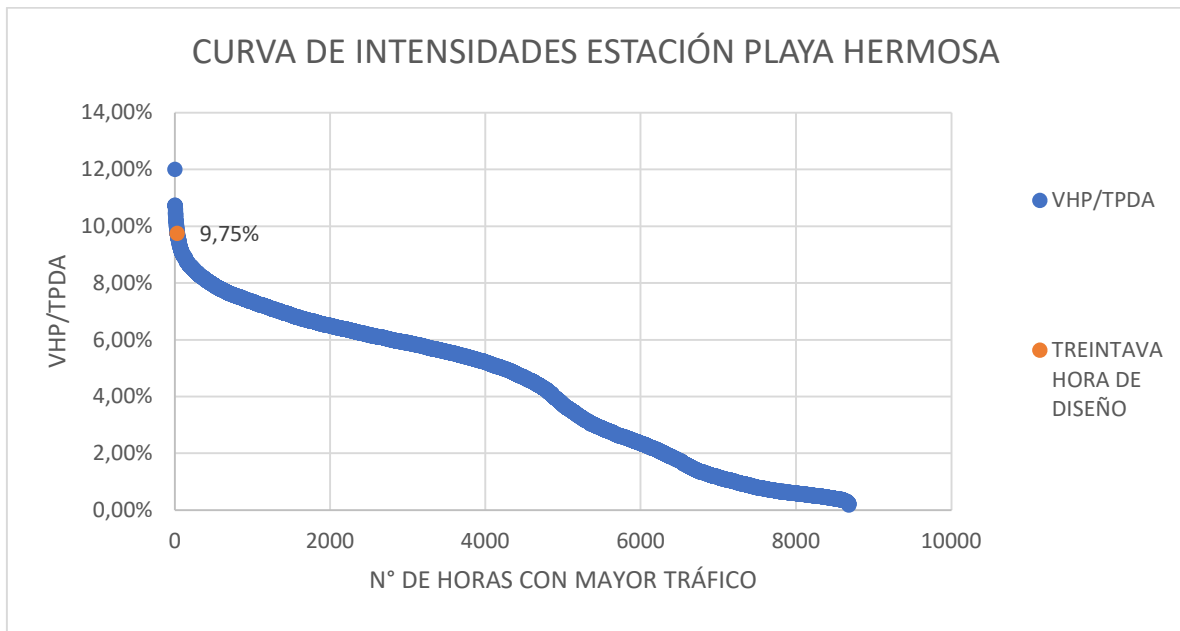
Gráfica 8: Curva de intensidades para obtención de Hora Treinta de Diseño de Estación Playa Hermosa
