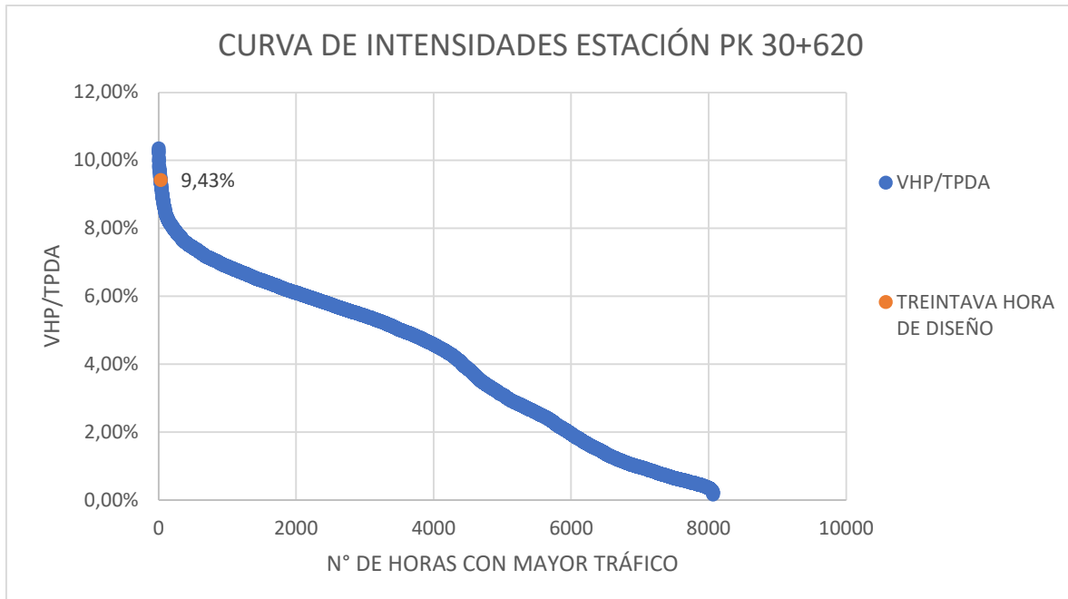
Gráfica 15: Curva de intensidades para obtención de Hora Treinta de Diseño de Estación 30+620
