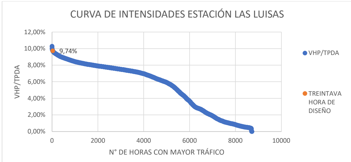
Gráfica 1: Curva de intensidades para obtención de Hora Treinta de Diseño de Estación de Las Luisas
