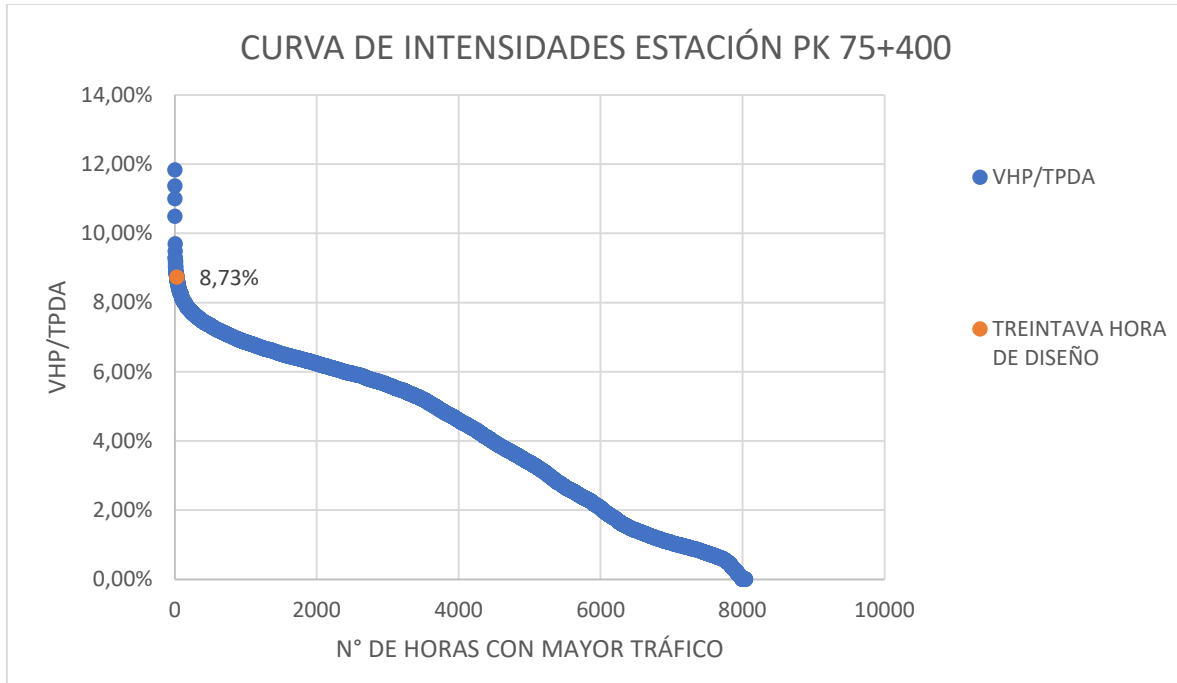
Gráfica 21: Curva de intensidades para obtención de Hora Treinta de Diseño de Estación 75+400
