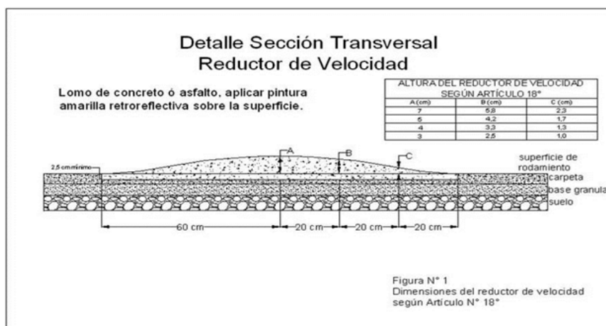
Figura N° 9. Corte típico de reductor tipo lomo
