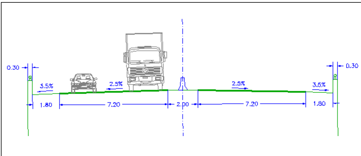
Figura 3.1. Esquema de la sección típica del viaducto
