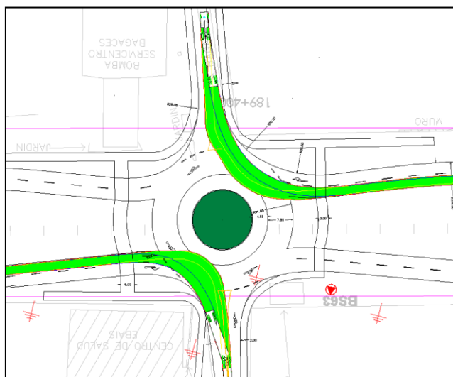
Figura N° 3.4. Esquema de circulación del tránsito en la rotonda y su diseño geométrico.
