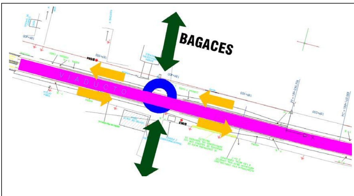
Figura N° 3.3. Esquema de flujos en el Paso a Desnivel Bagaces.
